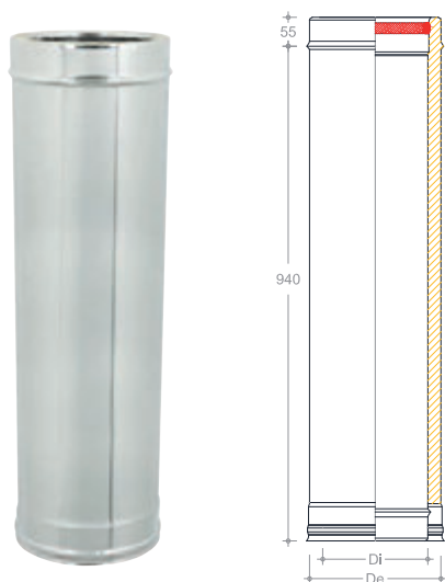
Art. LNIZDL100 - Module Linéaire 1000 mm
